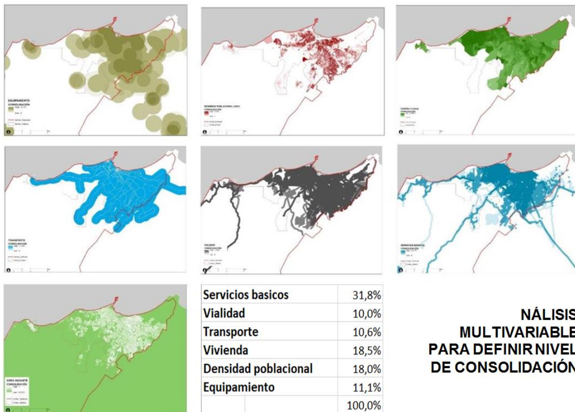
Gráfico N° 2 Análisis Multivariable
