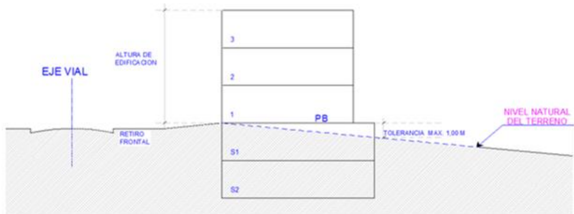
Gráfico N° 13 Edificaciones Sobre Plataformas Aterrazadas: con Pendiente Negativa
