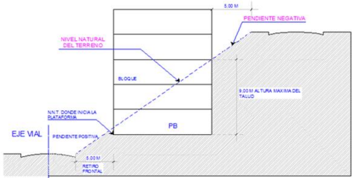
Gráfico N° 11 Edificaciones en Pendiente Positiva o Negativa Sobre Plataformas Aterrazadas
