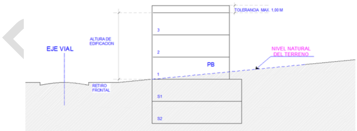
Gráfico N° 12 Edificaciones Sobre Plataformas Aterrazadas: con Pendiente Positiva
