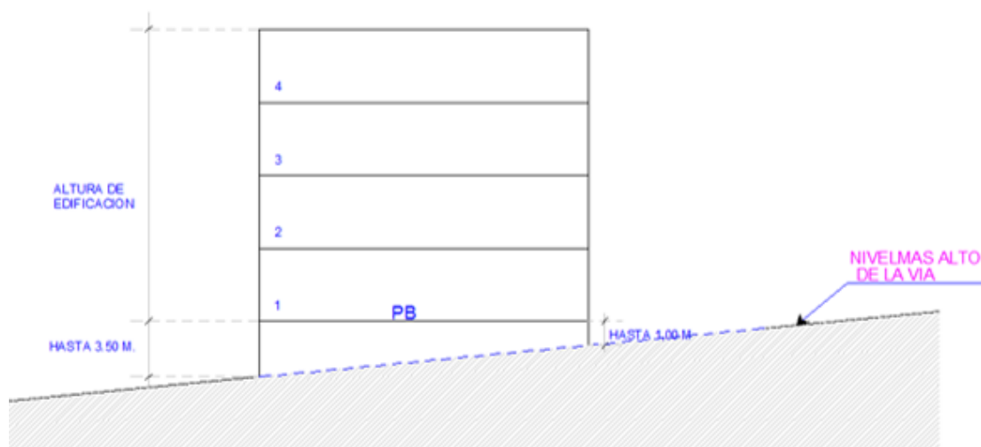
Gráfico N° 17 Edificaciones Aterrazadas
