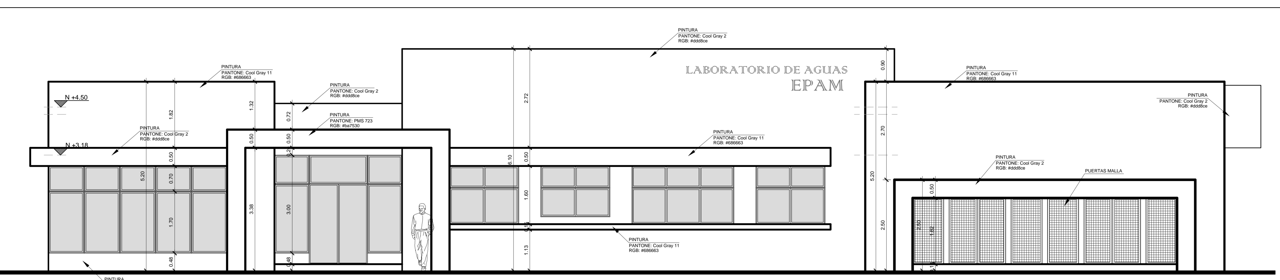
FACHADA OESTE
