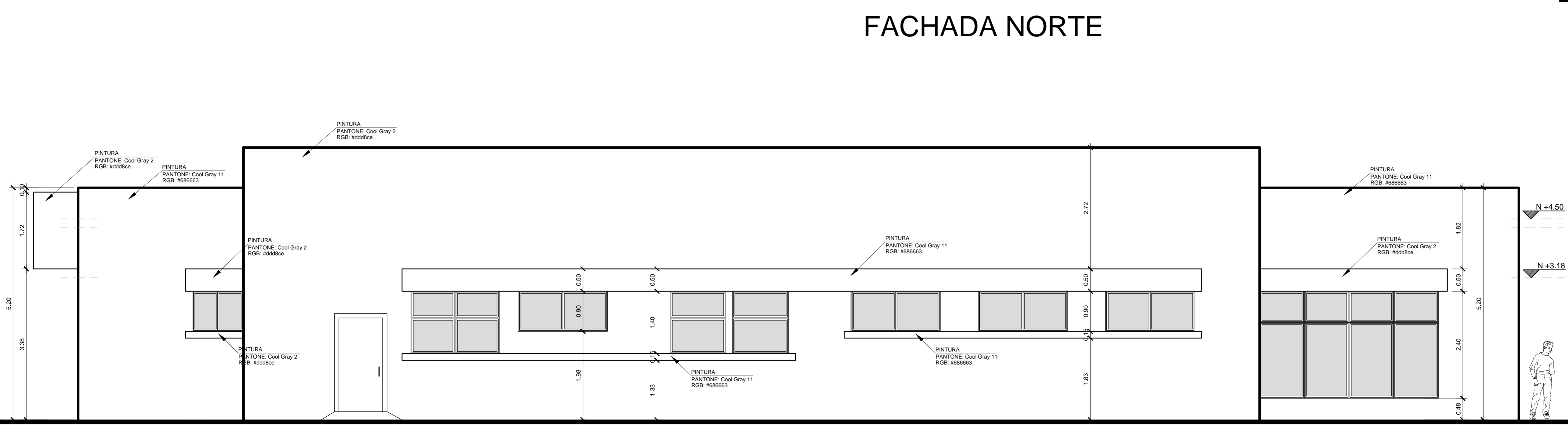
FACHADA ESTE
